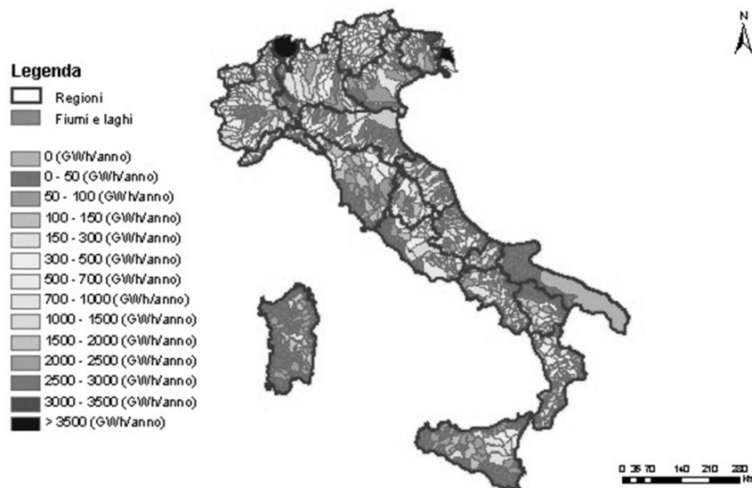
Figura 1 - Mappa del massimo potenziale idroelettrico ( fonte: [8])
