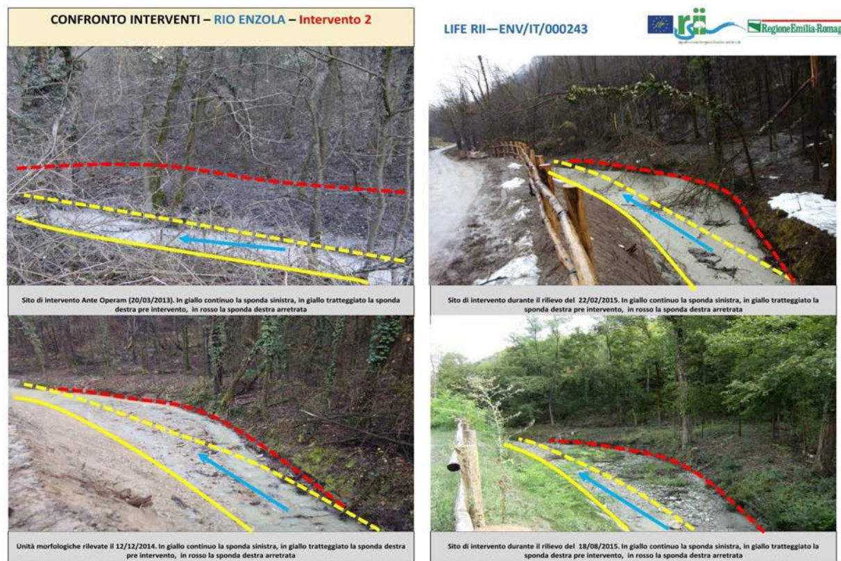
Figura 39 – Evoluzione morfologica dell'intervento “Allargamento di sezione”
