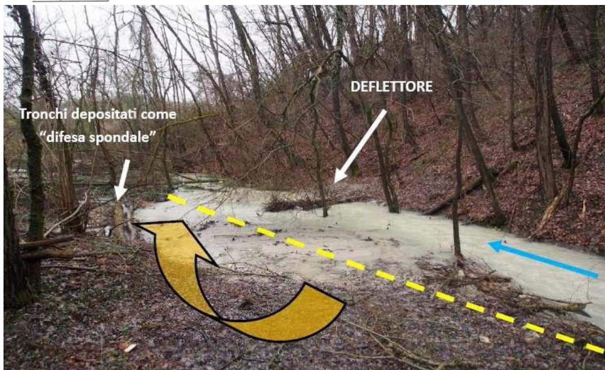
Figura 58 – Schema di massima e foto che illustra il funzionamento di un deflettore di corrente realizzato per l'aumento delle dinamiche laterali e dell'erosibilità della sponda opposta sul rio Bertolini.
