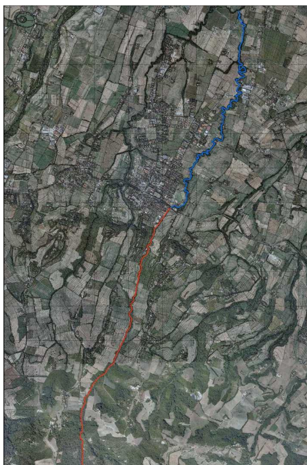
Figura 19 – Segmenti fisiografici del Rio Lavezza: collinare confinato (rosso); alta pianura (blu)
