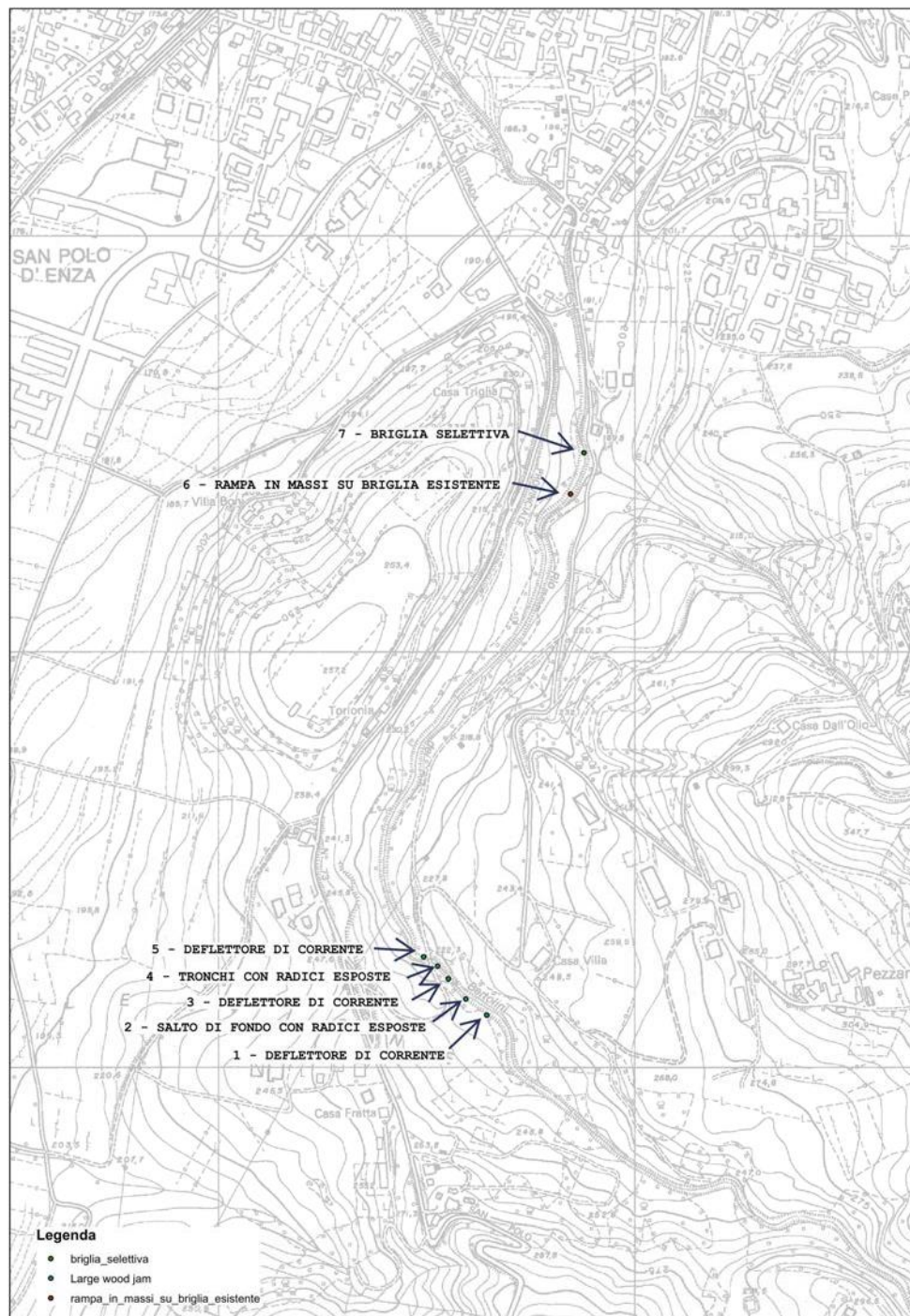
Figura 9 - Siti di intervento lungo il Rio Bertolini
