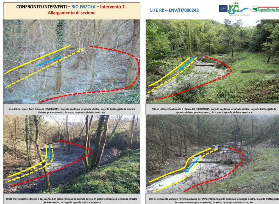
Figura 38 –Evoluzione morfologica dell'intervento "Allargamento di sezione"
