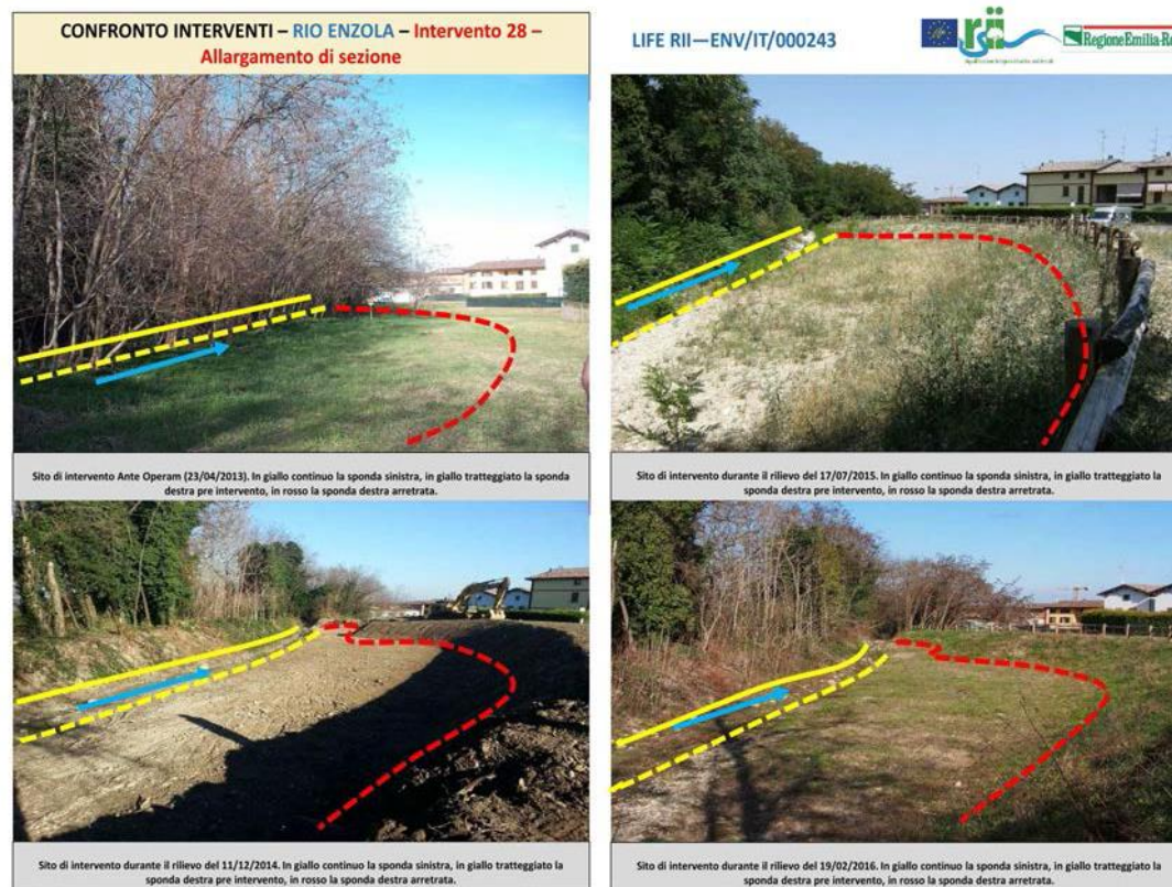
Figura 45 –Evoluzione morfologica dell'intervento “Allargamento di sezione”
