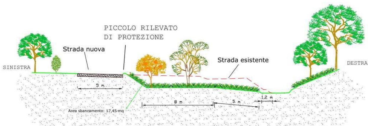
Figura 37 - Schema progettuale di un allargamento di sezione tipo
