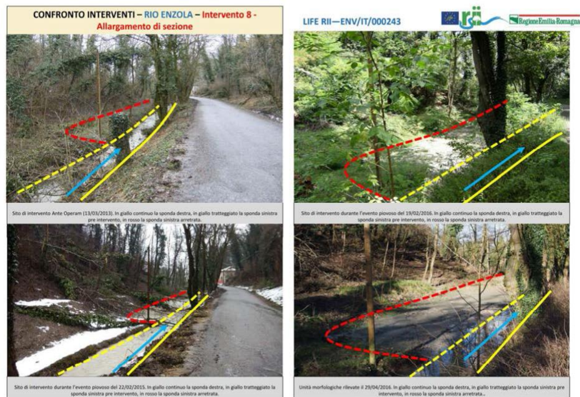
Figura 41 –Evoluzione morfologica dell'intervento “Allargamento di sezione”
