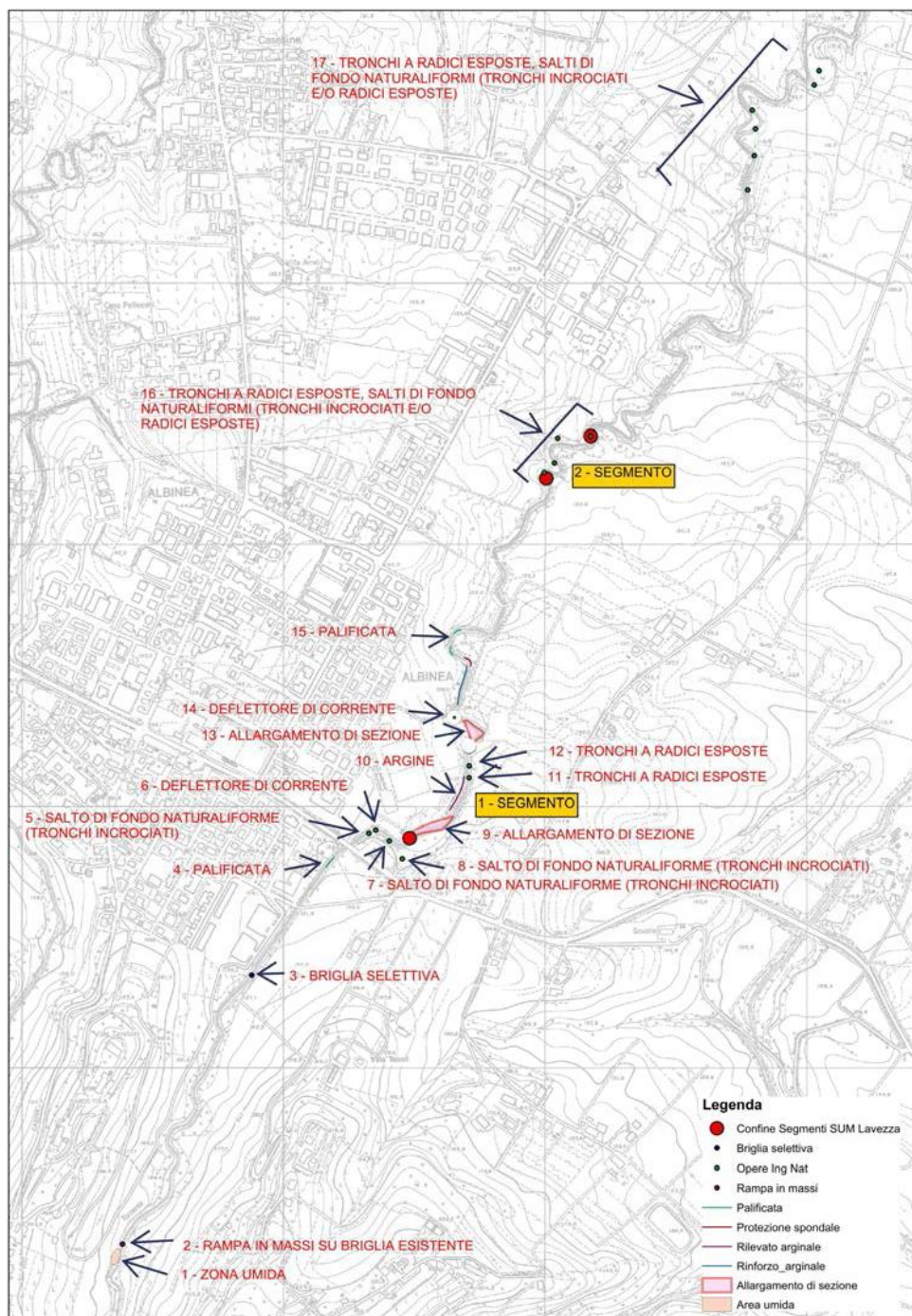
Figura 5 - Siti di intervento lungo il Rio Lavezza (in giallo sono indicati anche i segmenti analizzati con l'indice SUM)
