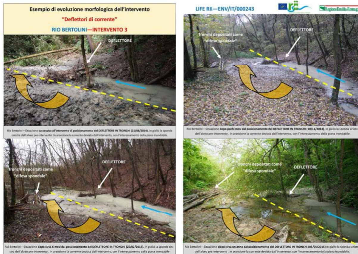
Figura 59 –Evoluzione morfologica dell'intervento "Deflettori di corrente"
