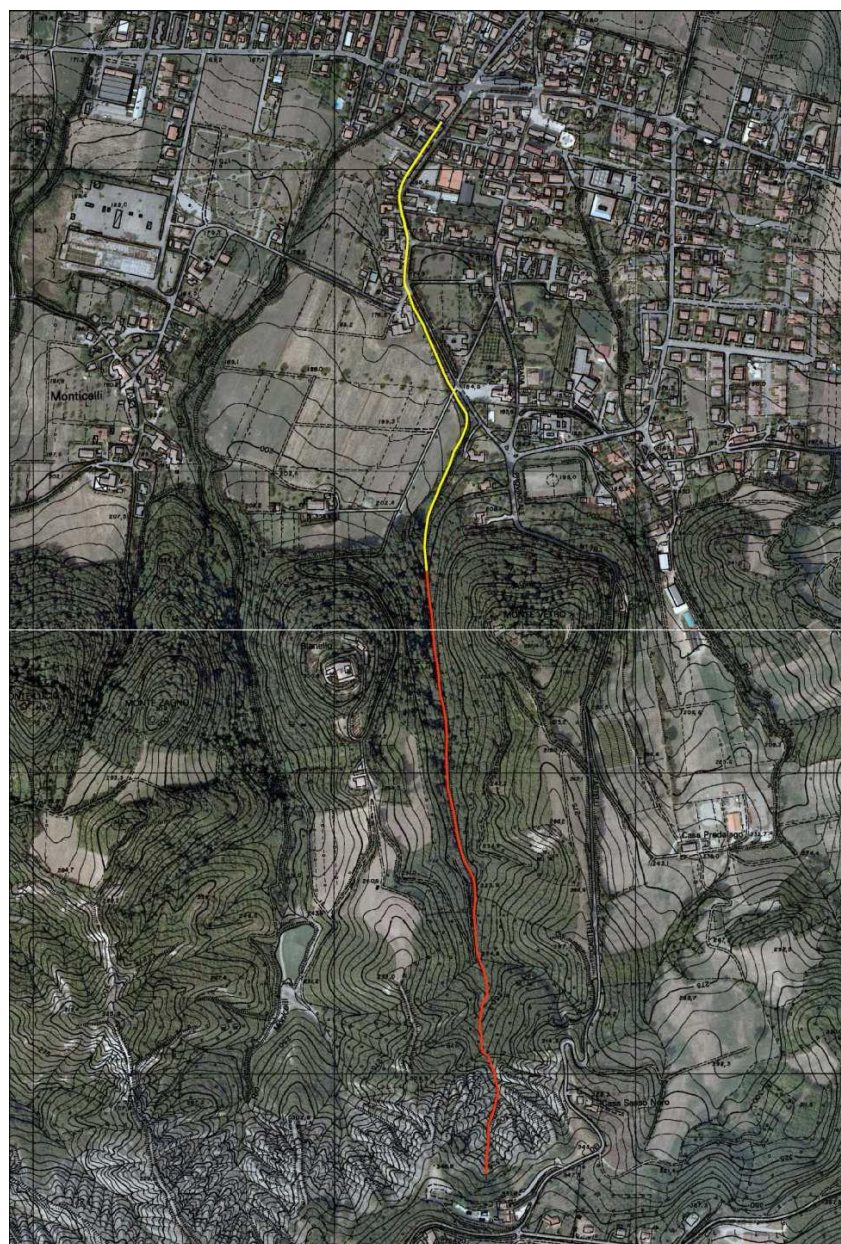
Figura 17 – Morfologie fluviali presenti nel Rio Bianello: confinato a canale singolo (rosso) e sinuoso (giallo).
