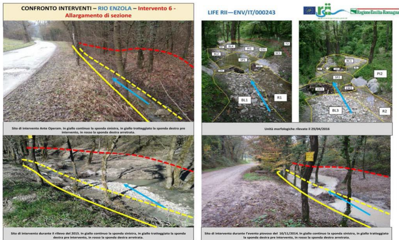
Figura 40 –Evoluzione morfologica dell'intervento “Allargamento di sezione”
