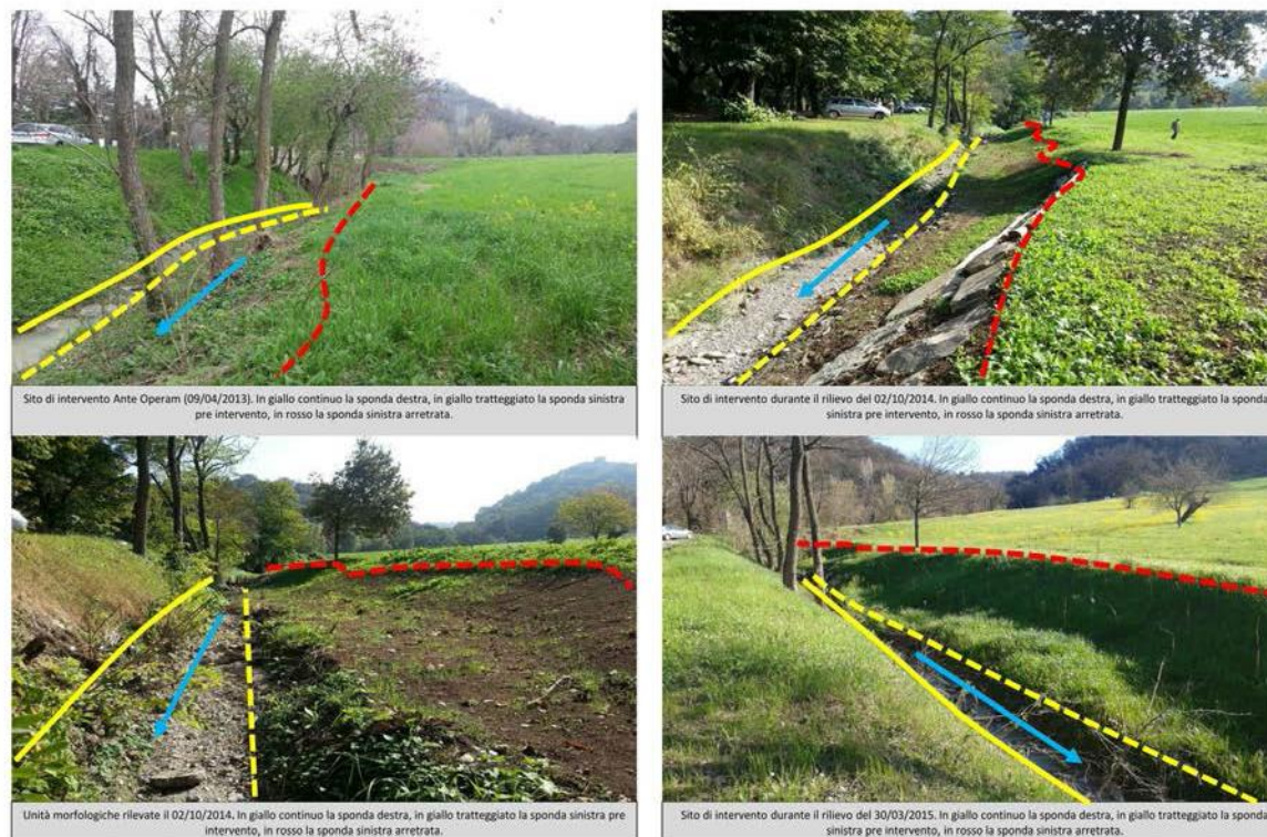
Figura 48 –Evoluzione morfologica dell'intervento "Allargamento di sezione"
