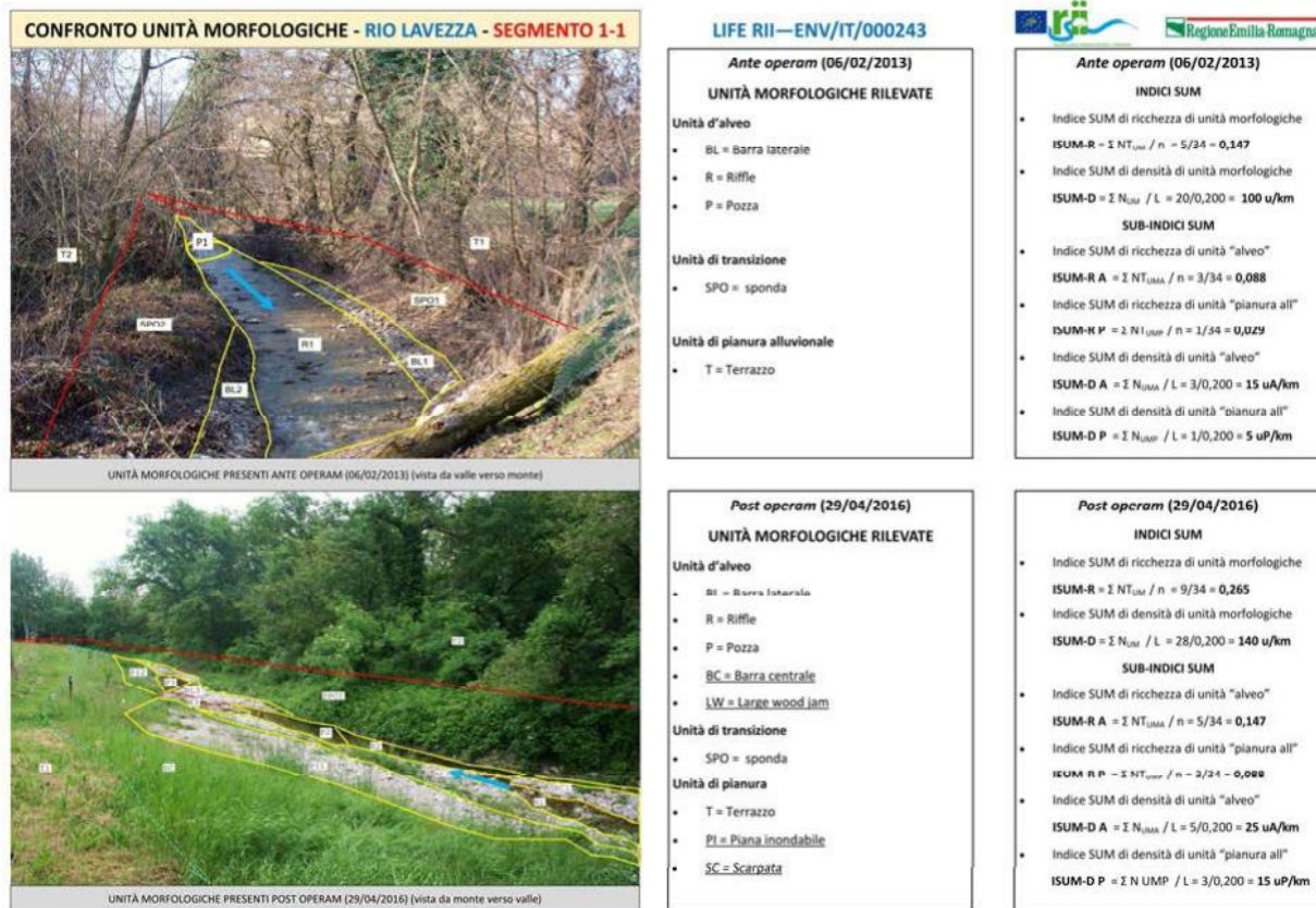
Figura 33 –Rio Lavezza – Segmento 1 - Calcolo di alcuni indici SUM
