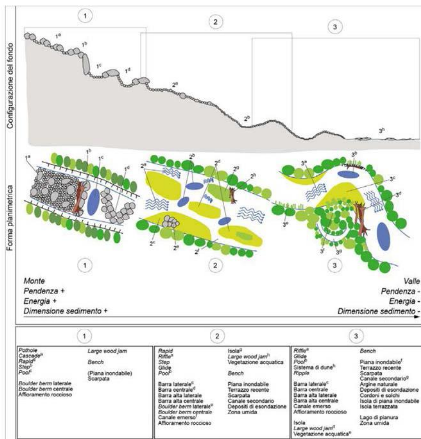
Figura 23 – Distribuzione delle unità morfologiche da monte verso valle
