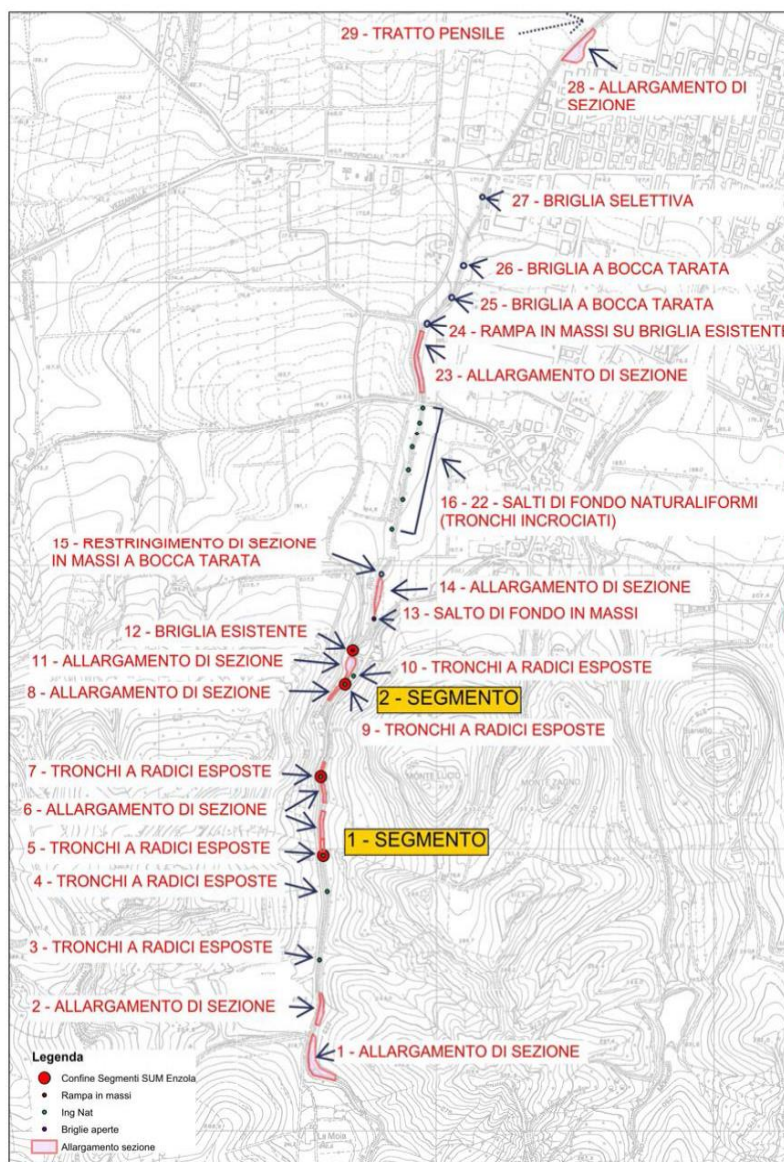
Figura 1 - Siti di intervento lungo il Rio Enzola (in giallo sono indicati anche i segmenti analizzati con l'indice SUM)
