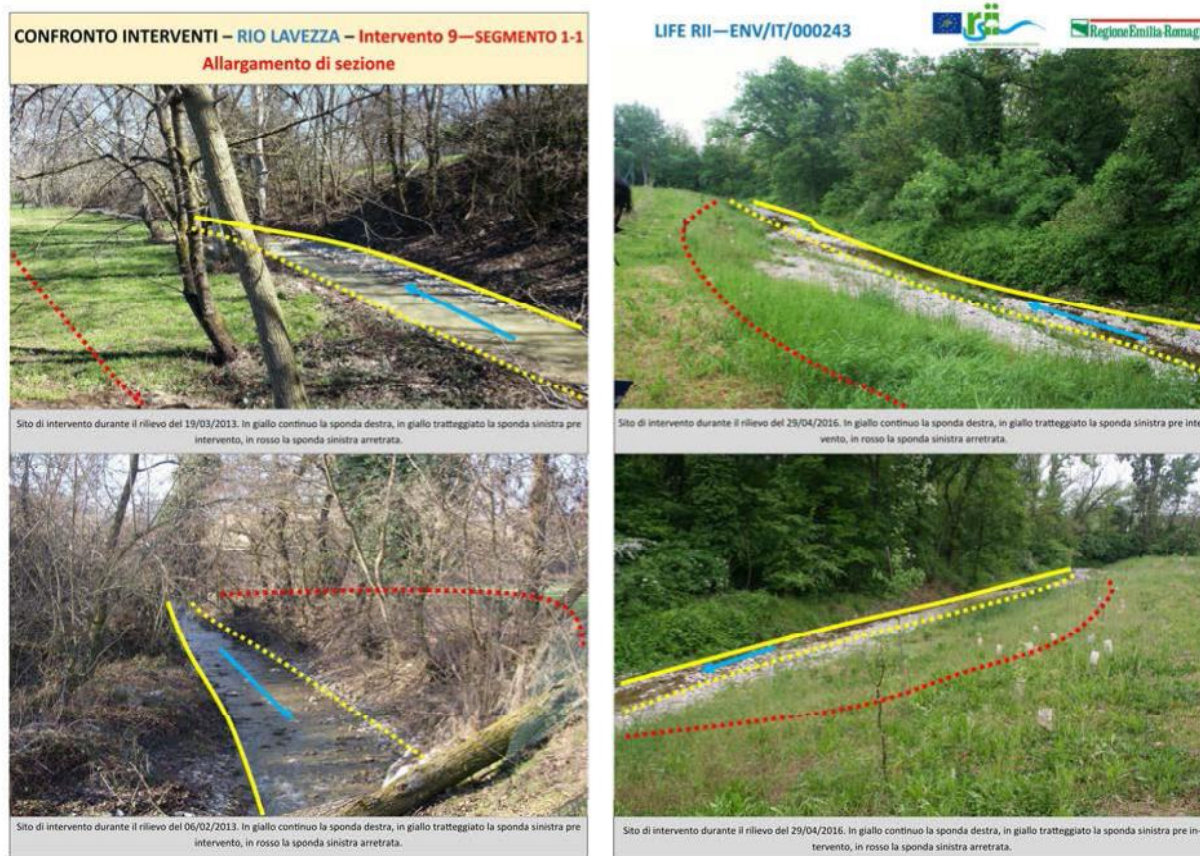
Figura 50 -- Evoluzione morfologica dell'intervento “Allargamento di sezione”
