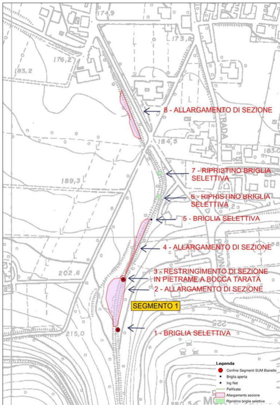
Figura 3 - Siti di intervento lungo il Rio Bianello (in giallo sono indicati anche i segmenti analizzati con l'indice SUM)
