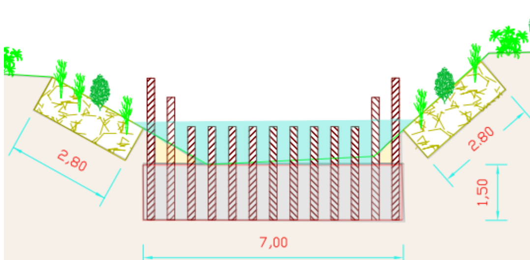
Figura 4 – Sezione di massima dell'intervento. La briglia selettiva nella configurazione a pettine permette di intercettare i materiali di grandi dimensioni (Fonte: Consorzio di bonifica dell'Emilia Centrale)
