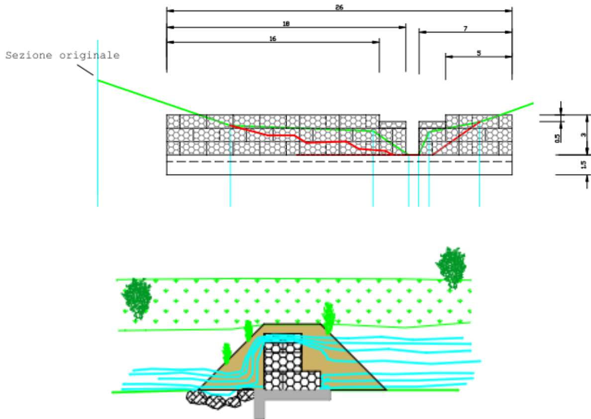
Figura 3 – Schema del restringimento di sezione a bocca tarata con anima in pietrame, che permette il passaggio delle portate ordinarie e dei sedimenti e genera un accumulo delle acque a monte dello stesso in caso di piena. In alto, vista in pianta, al centro vista in sezione trasversale, in basso vista in sezione longitudinale.
