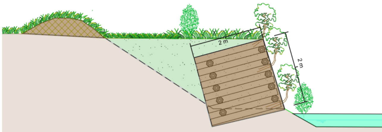
Figura 5 – Schema di massima dell’intervento. (Fonte: Foto Monaci Marco (a sinistra); Regione Emilia-Romagna, 2012. Linee guida per la riqualificazione ambientale dei canali di bonifica in Emilia-Romagna (a destra); Regione Lazio. Manuale settore idraulico. Scheda 025 – Palificata viva spondale (a destra) ).
