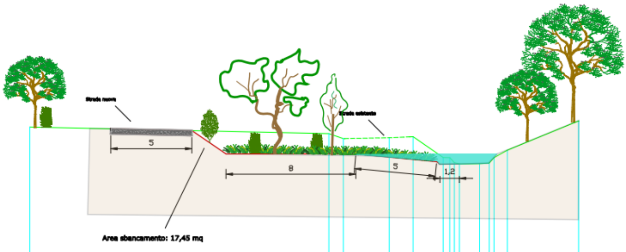
Figura 9 - Schema di massima di un intervento di sbancamento, abbassamento e riquilificazione dell'alveo nel tratto montano, nell'area posta nei pressi di una ex cava.
