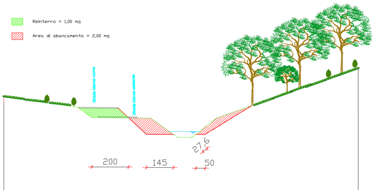
Figura 10 - Schema di massima di un intervento di sbancamento, abbassamento e riquilificazione dell'alveo nel tratto collinare, in corrispondenza di una strada sterrata esistente posta su aree demaniali.
