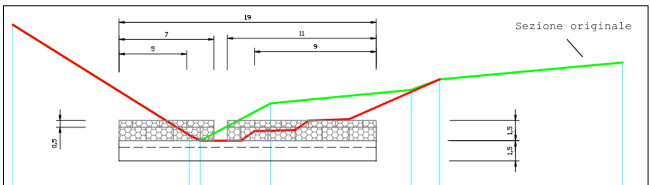
Figura 12 – Schema del restringimento di sezione a bocca tarata con anima in pietrame previsto nell’area privata (pianoro) posto in corrispondenza di un allargamento di sezione: l’intervento permette il passaggio delle portate ordinarie e dei sedimenti e genera un accumulo delle acque a monte dello stesso in caso di piena. In alto, l’intervento visto in pianta (a sinistra) e in sezione longitudinale all’alveo. In basso l’intervento visto in sezione trasversale all’alveo
