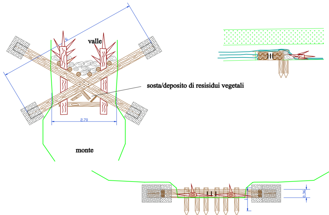
Figura 14 – Schema tipologico dell'intervento. La costruzione di un piccolo salto di fondo in tronchi, massi e radici esposte permette di innalzare il livello idrico a monte e aumentare così la frequenza di allagamento delle aree golenali limitrofe, garantendo inoltre la diversificazione degli habitat in alveo. (Tratto e rielaborato da: Washington Departments of Fish and Wildlife, Natural Resources, Transportation and Ecology et al, 2012. Stream Habitat Restoration Guidelines e Ministry of environment, lands and parks – British Columbia, 1997. Fish habitat rehabilitation procedures. Watershed restoration technical circular n.9).
