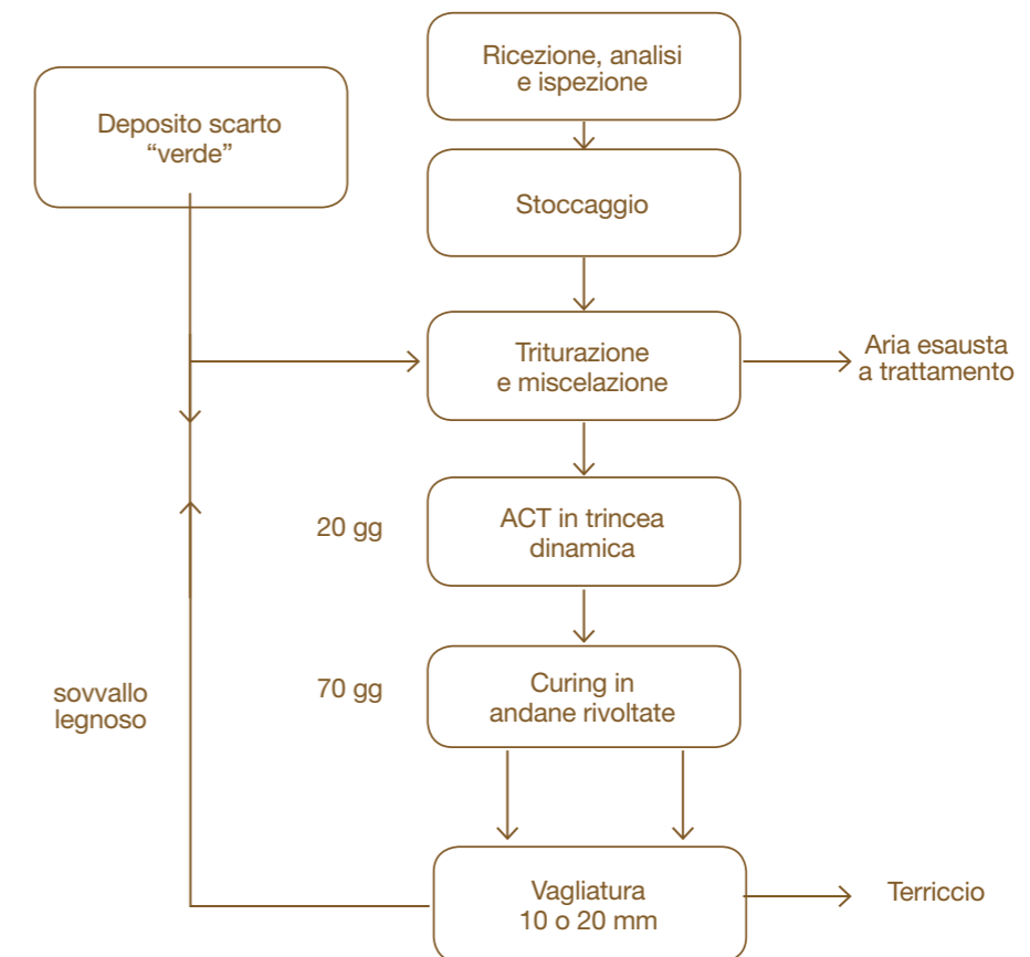
Figura 20. Schema di flusso di un impianto a tecnologia dinamica per il trattamento di biomasse ad elevata fermentescibilità
