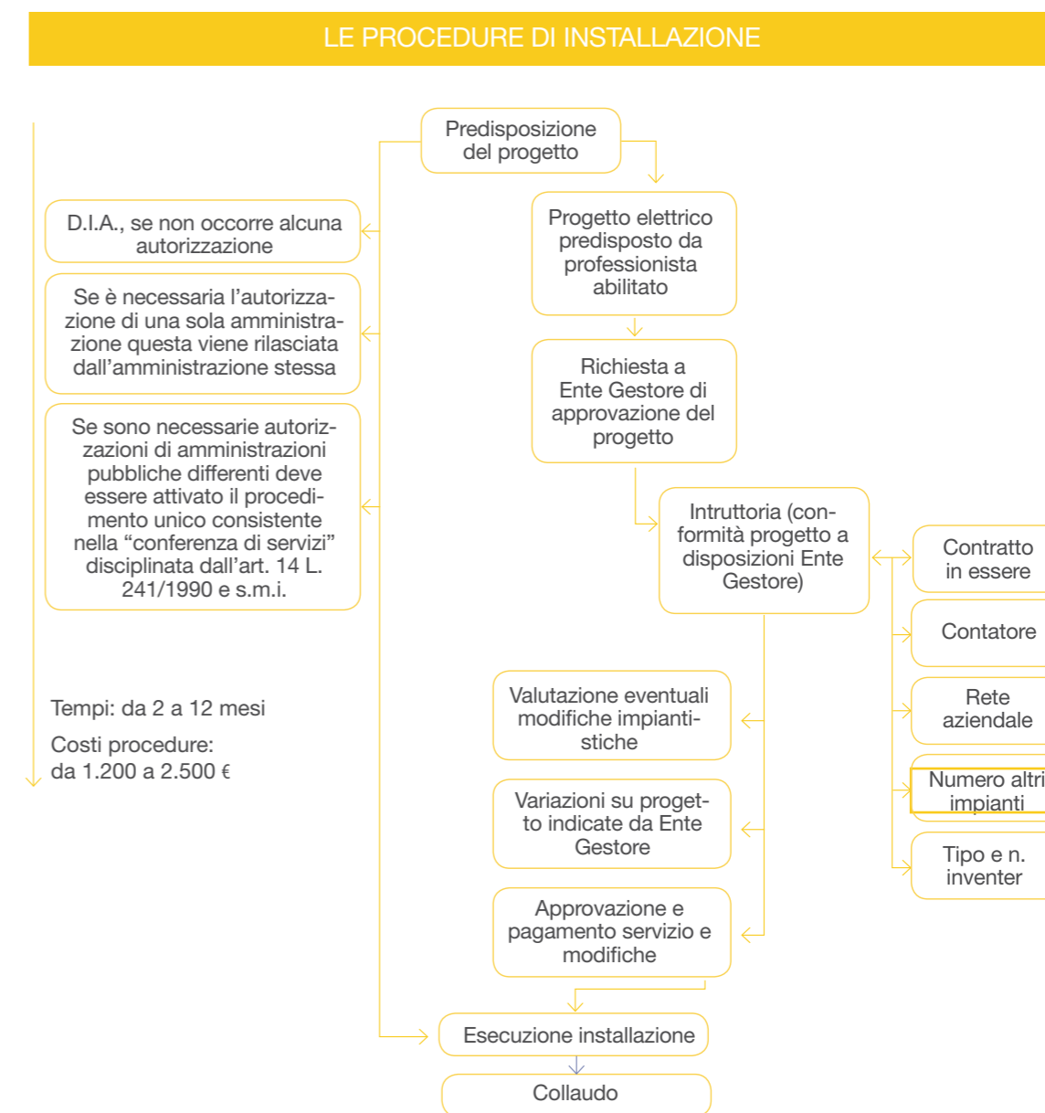
Figura 2. Schema di sintesi sulle procedure di installazione di un impianto fotovoltaico
