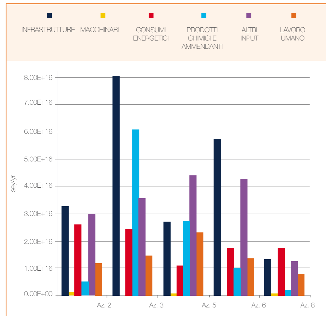
Figura 24. Bilancio energetico e contributo dei diversi elementi al totale energetico delle aziende analizzate
