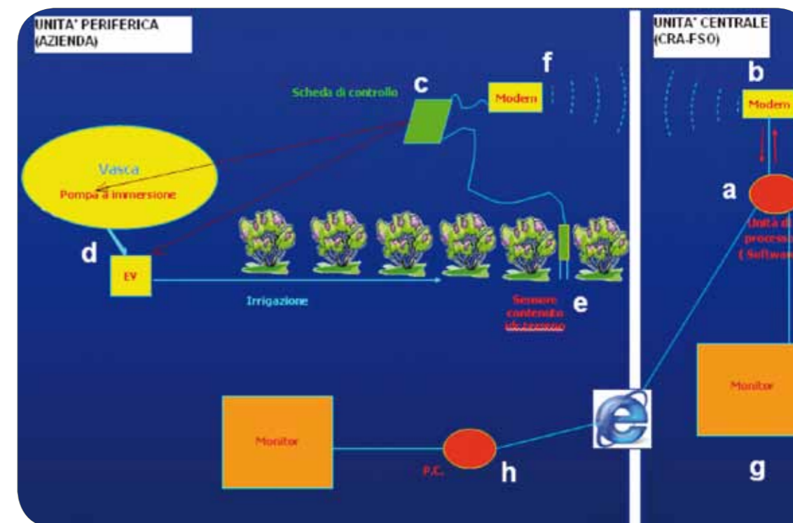
Figura 1. Schema di funzionamento del sistema di automazione irrigua
