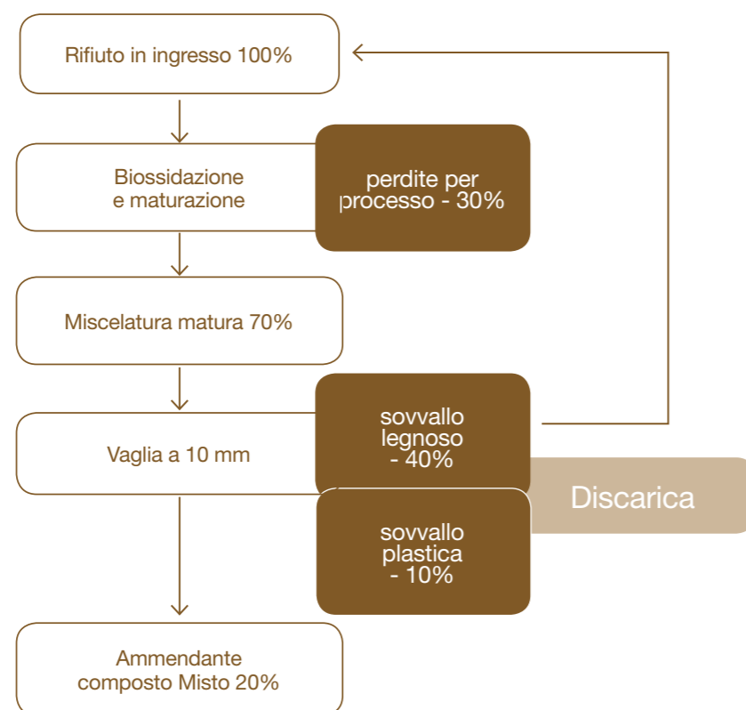
Figura 21. Bilancio di massa relativo ad un sistema per l'ottenimento di un ammendante compostato misto.
