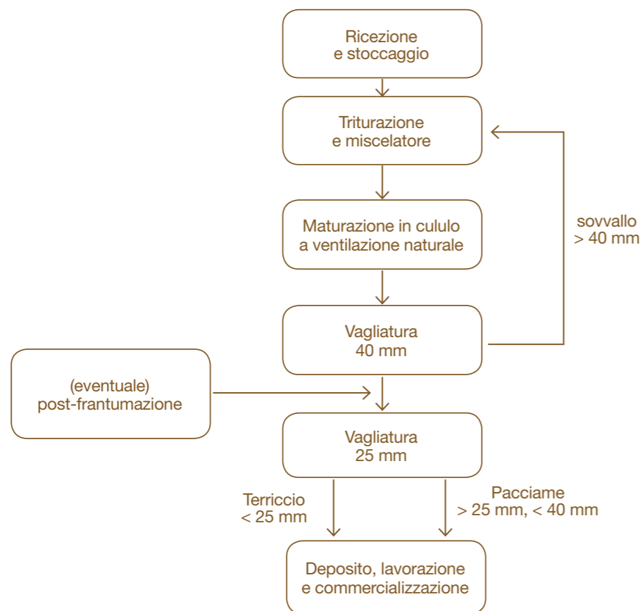
Figura 19. Schema operativo di un impianto industriale di compostaggio del "verde"
