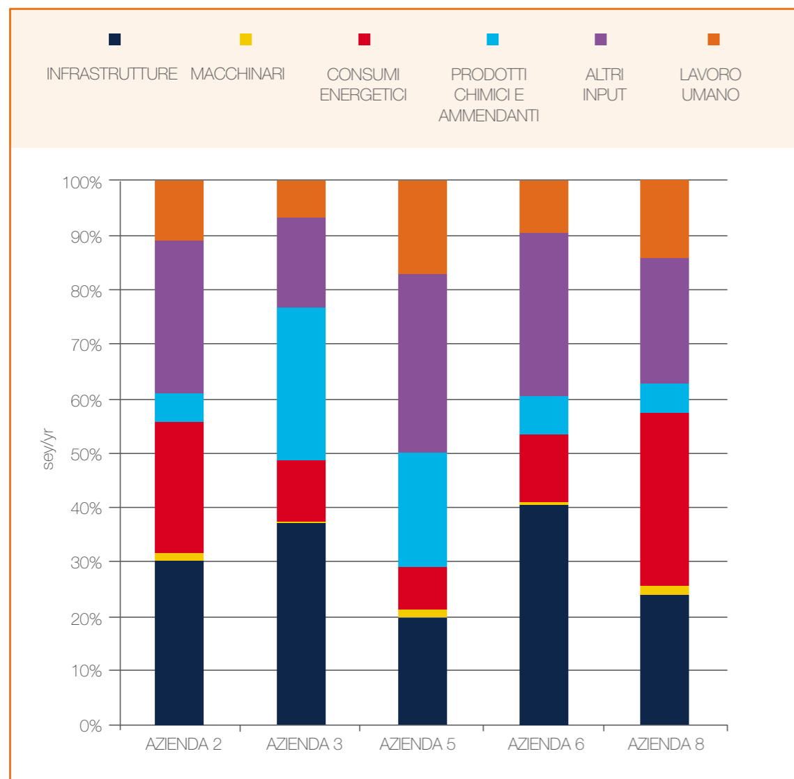
Figura 26. Bilancio energetico e contributo dei diversi elementi al totale energetico
